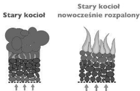
Rys. Kocioł zasypowy spalający przeciwprądowo vs kocioł zasypowy spalający współprądowo
